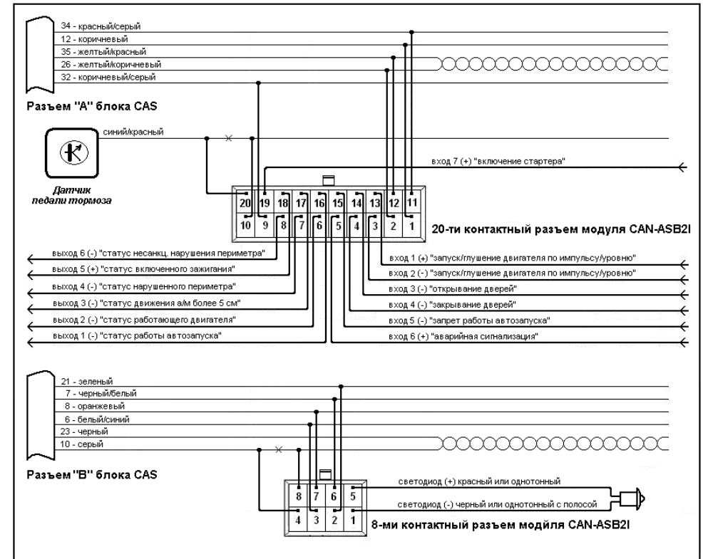
Рис. 1. Схема подключения модуля CAN-ASB21
